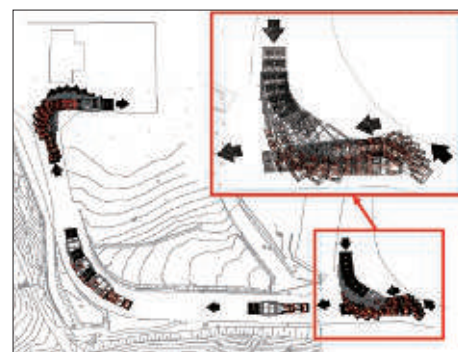
トレーラーの旋回軌跡図
