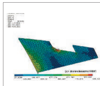
構造解析ソフトによる強度検証
